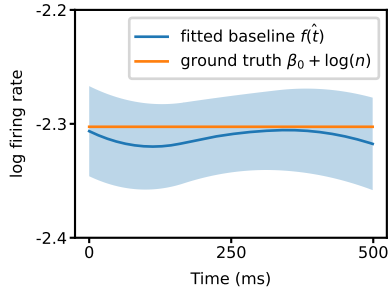
Population baseline
